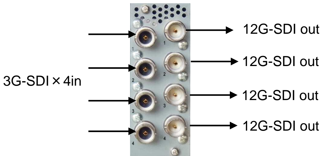
DUX-20 背面パネル
